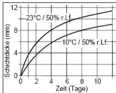
Diagramm 1: Durchhärtgeschwindigkeit für Sikaflex®-252
